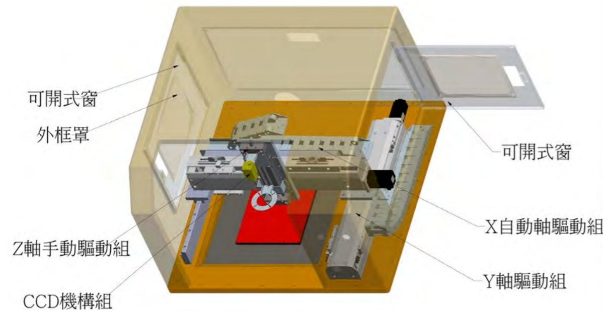
圖 1. 產品結構
